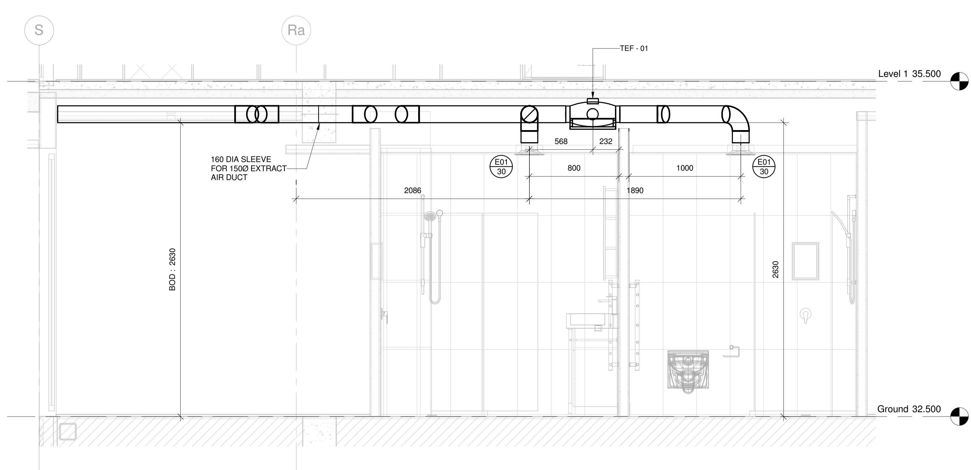
L SECTION L M117 SCALE : 1 : 20
