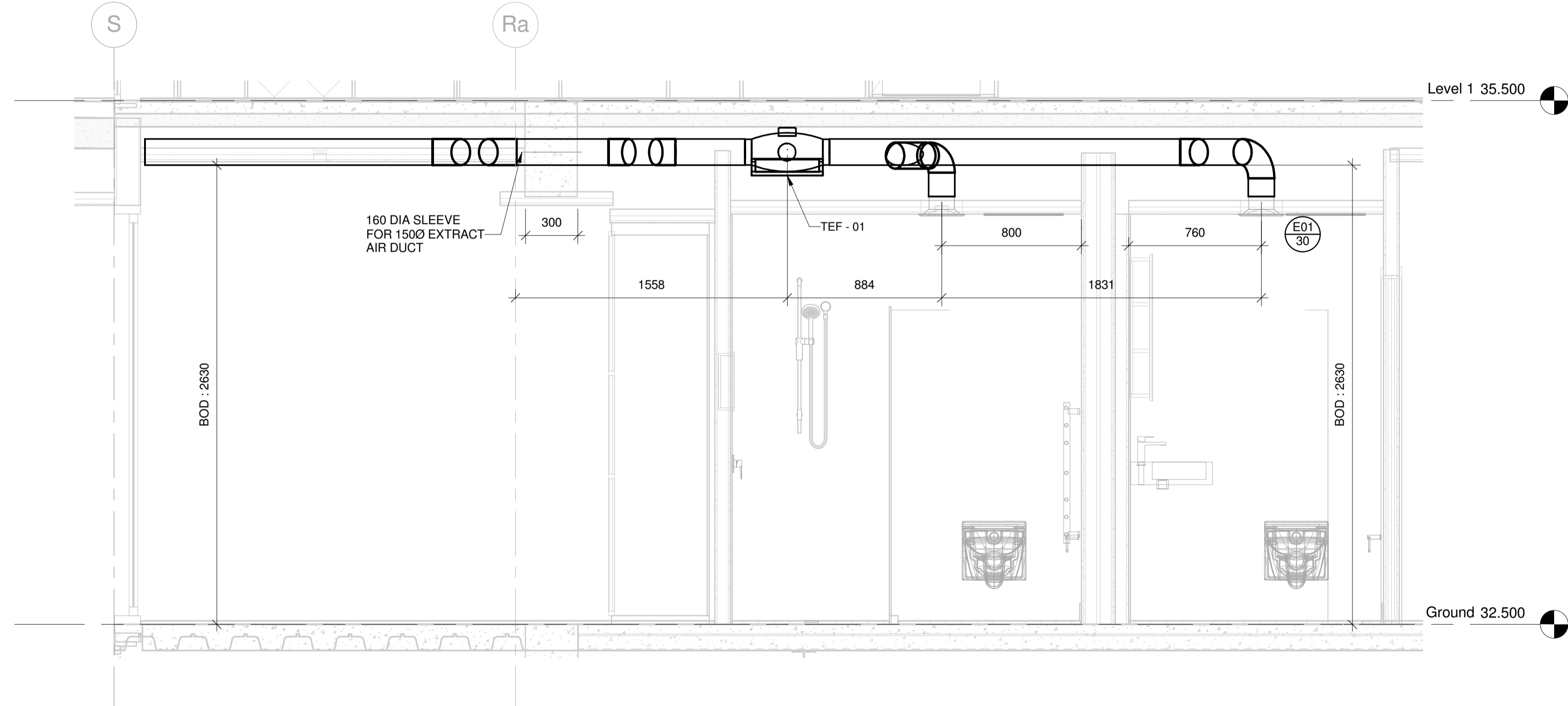
N SECTION N M117 SCALE : 1 : 20
