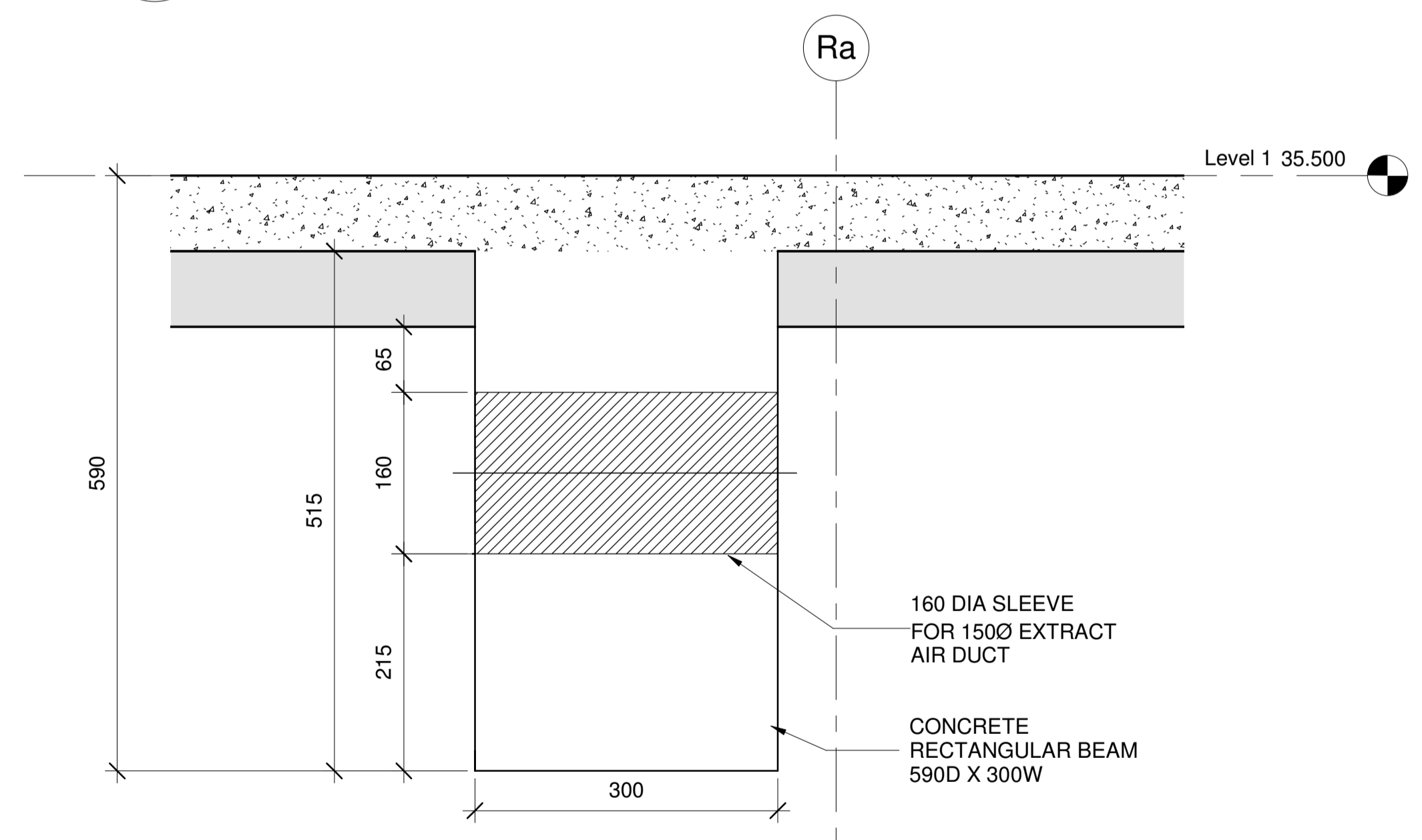
P SECTION P (TYP.) M118 SCALE : 1 : 5
