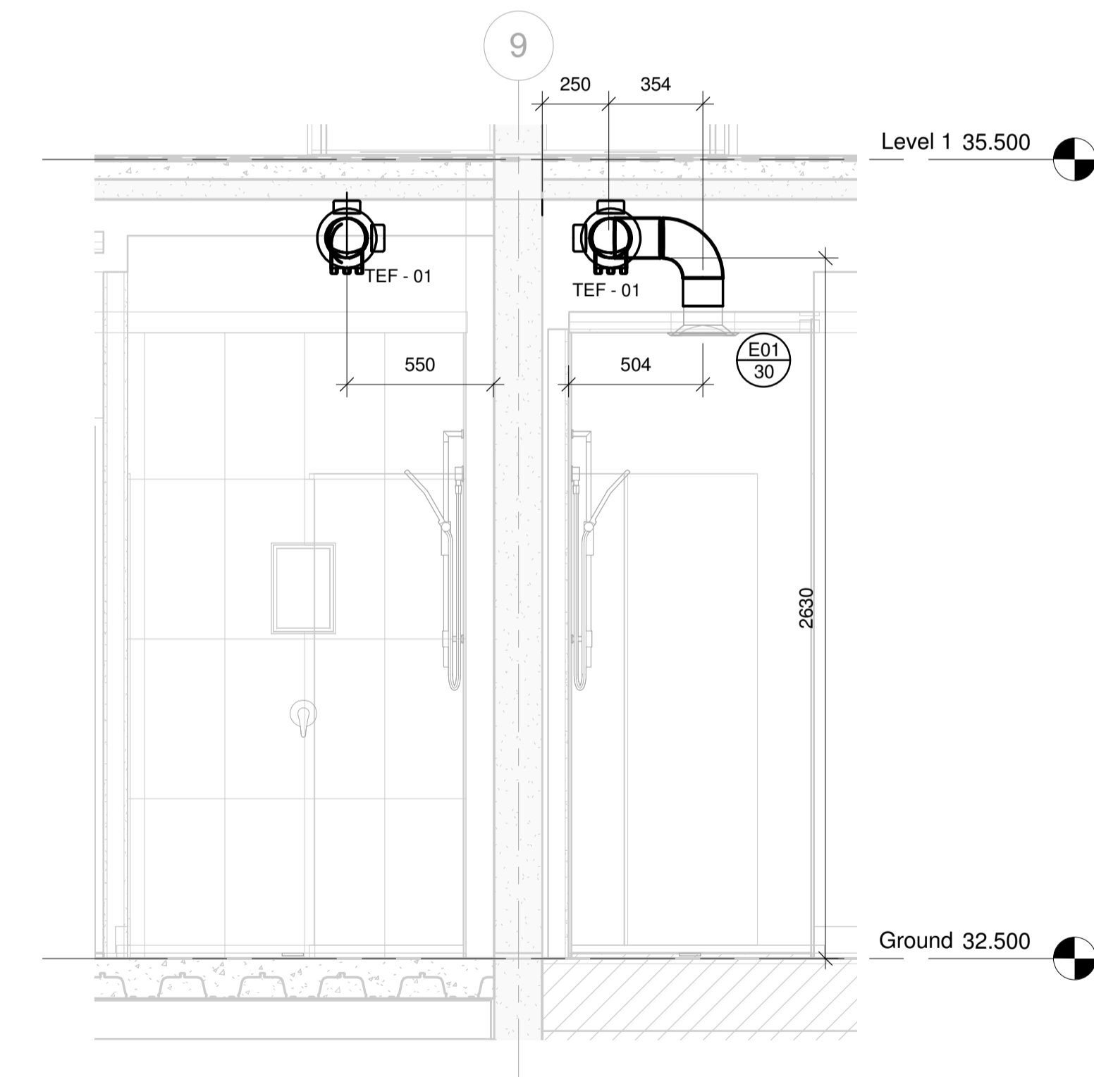
M SECTION M M117 SCALE : 1 : 20
