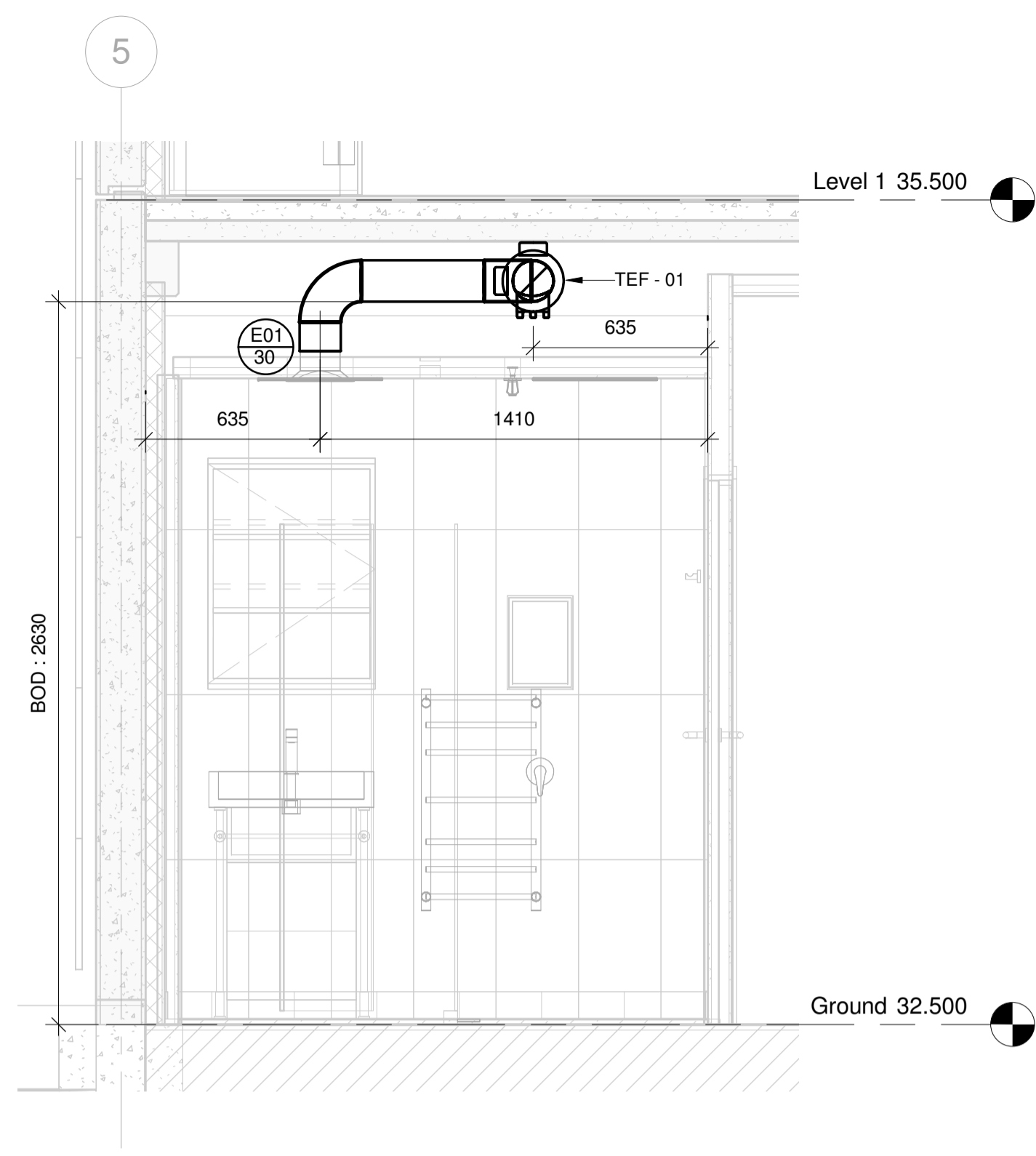
K SECTION K M117 SCALE : 1 : 20
