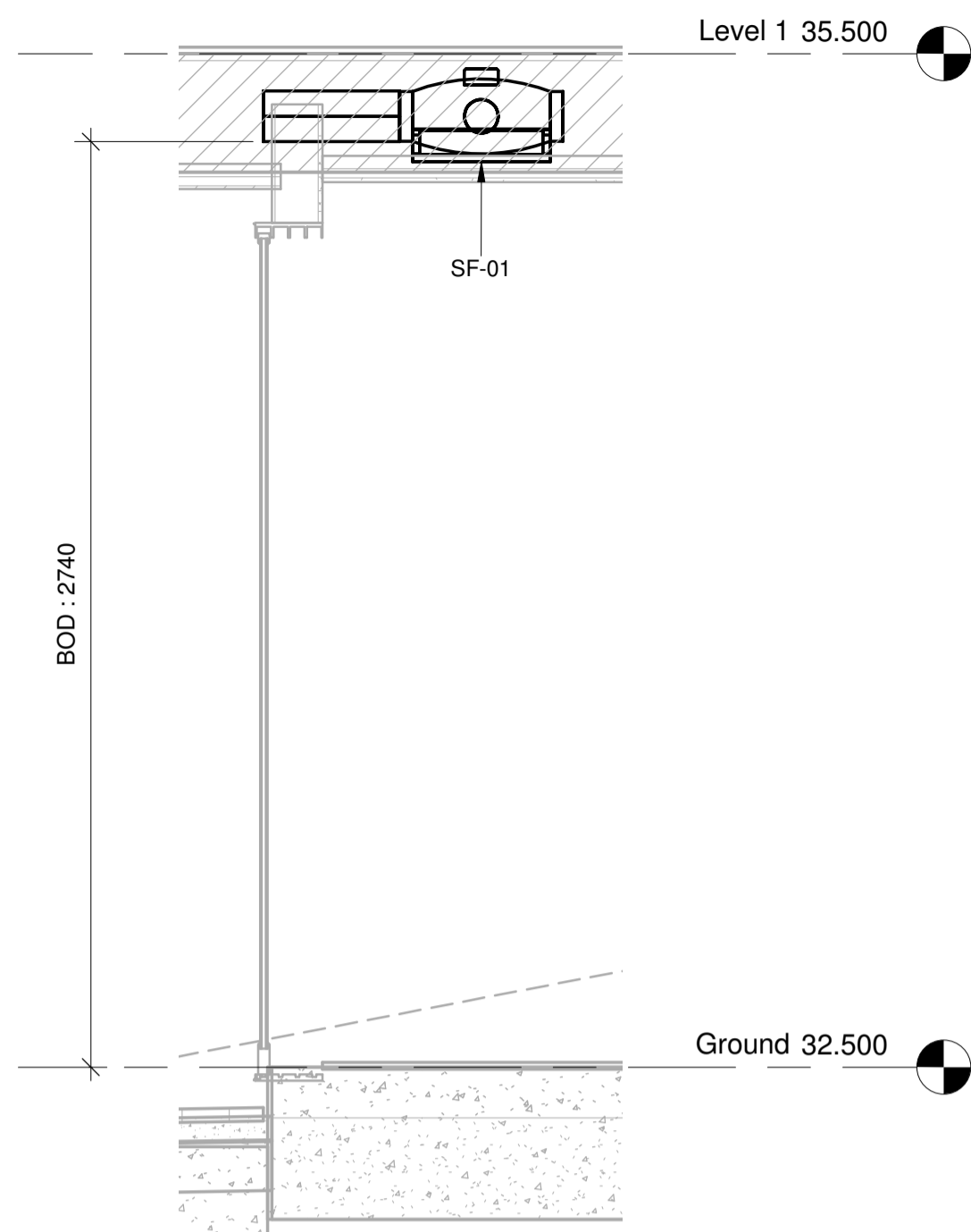
R SECTION R M120 SCALE : 1 : 20
