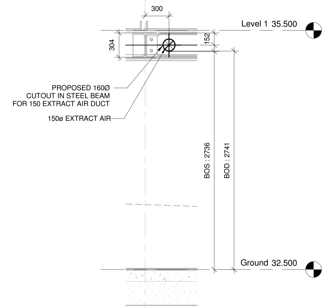
Q SECTION Q M119 SCALE : 1 : 25
