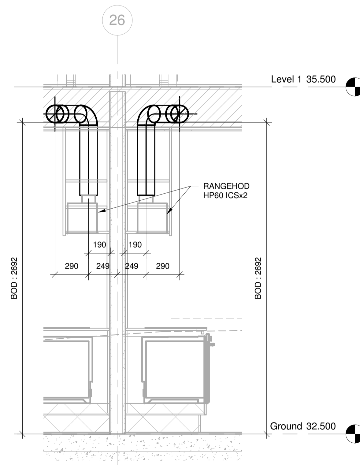
U SECTION U M120 SCALE : 1 : 20
