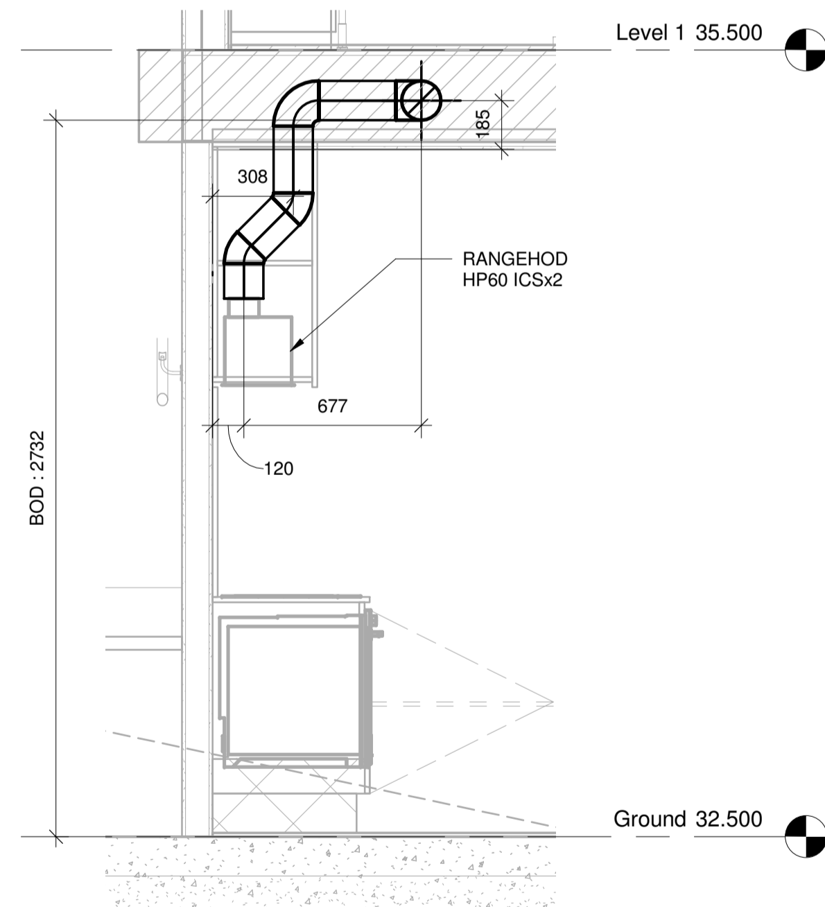
T SECTION T M120 SCALE : 1 : 20
