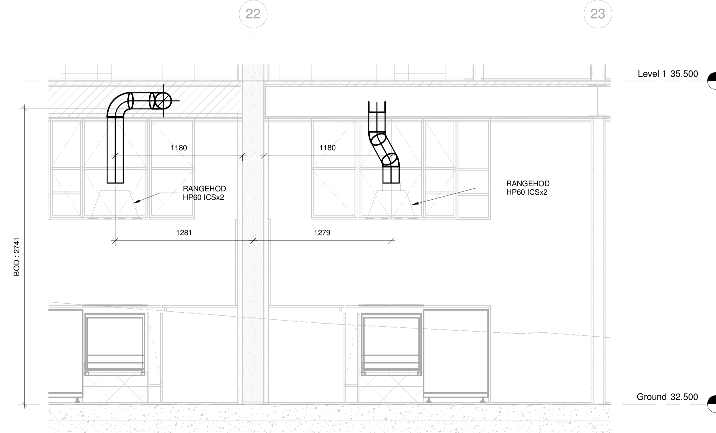
V SECTION V M120 SCALE : 1 : 20
